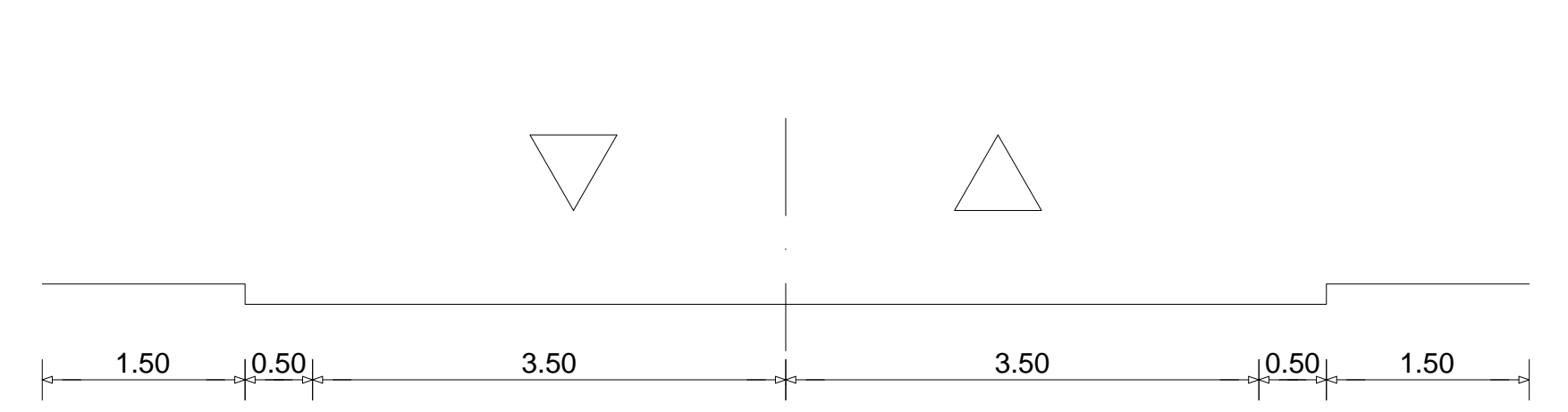
SEZIONE TIPO STRADA DI ACCESSO - scala 1:50
