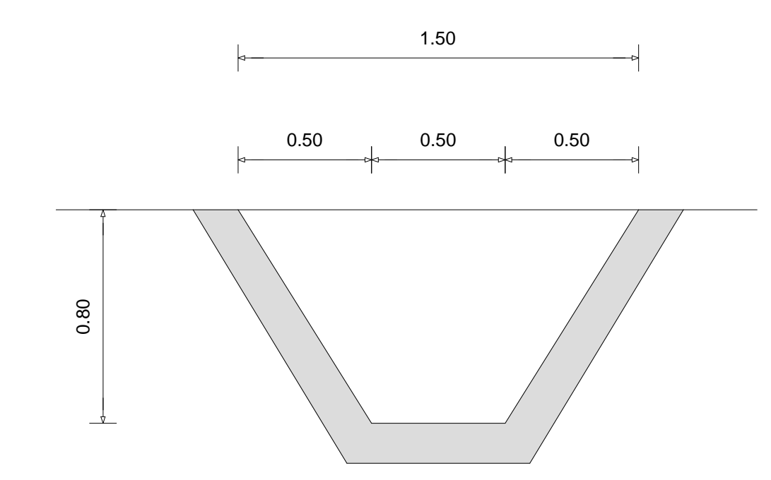
SEZIONE TIPO CUNETTA - scala 1:20
