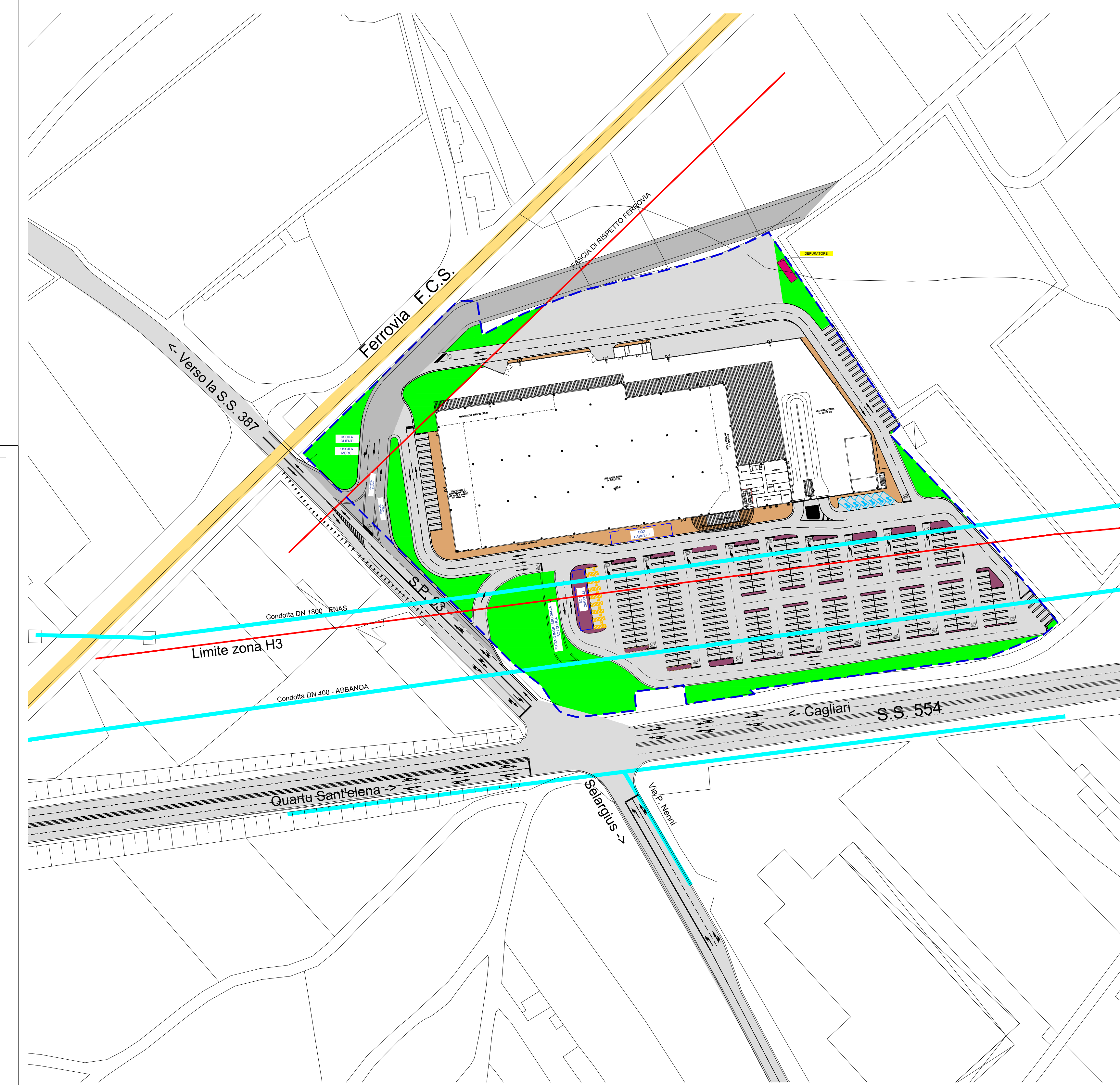
ACCESSO AL LOTTO DA VIABILITA' ATTUALE - scala 1:1.000
