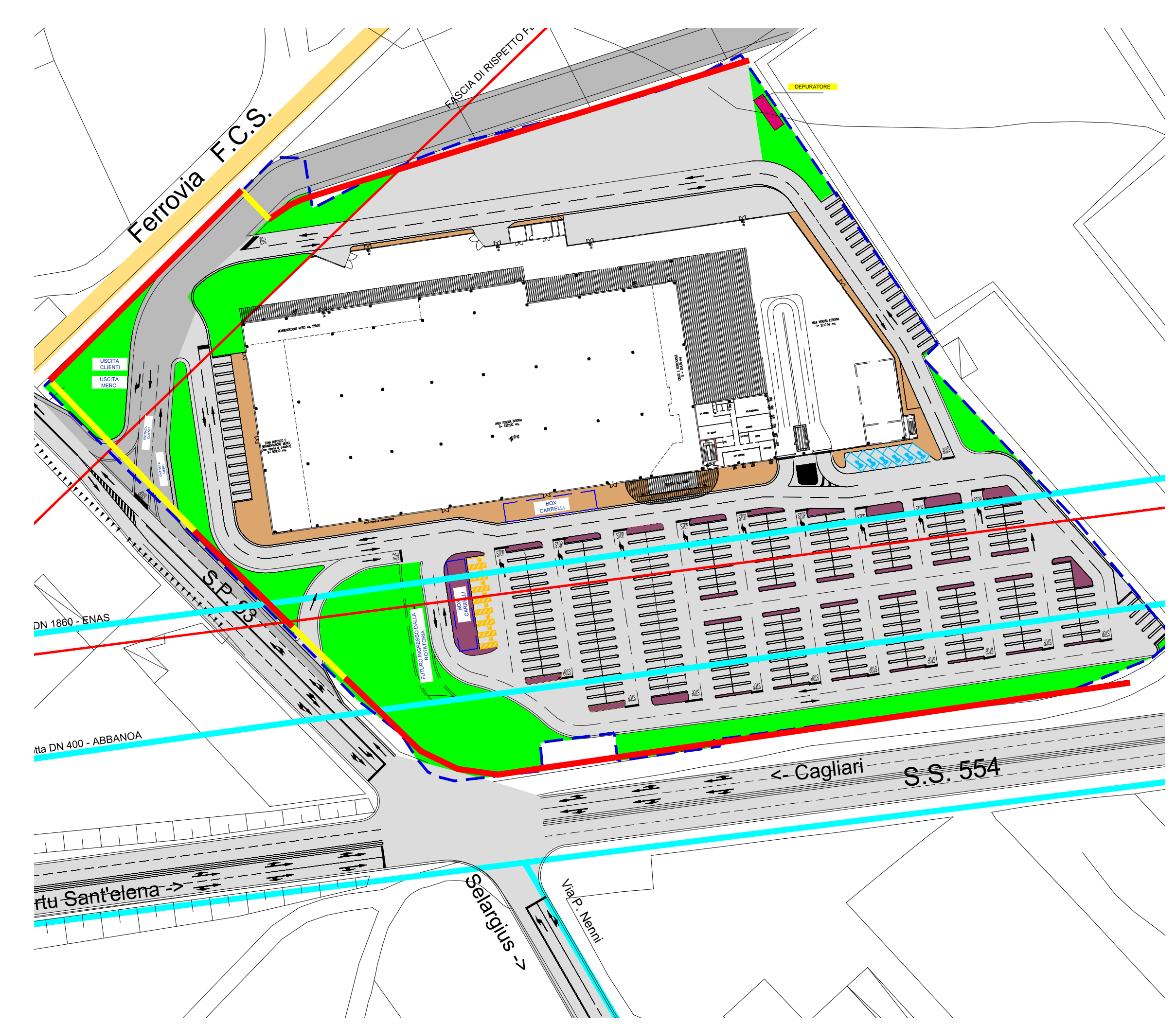
SCHEMA RACCOLTA ACQUE METEORICHE - scala 1:1.000
